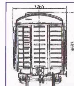
ГРУЗОВОЙ ВАГОН
