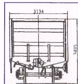
ГРУЗОВОЙ ПОЛУВАГОН
